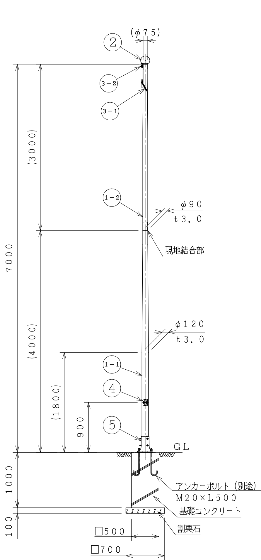
ポール姿図 S=1:40
