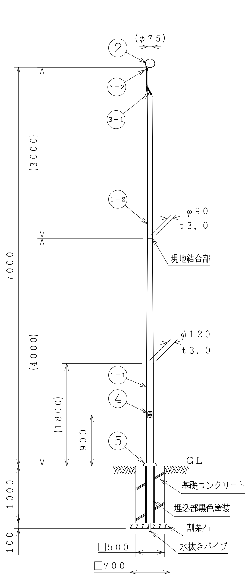
ポール姿図 S = 1 : 40
