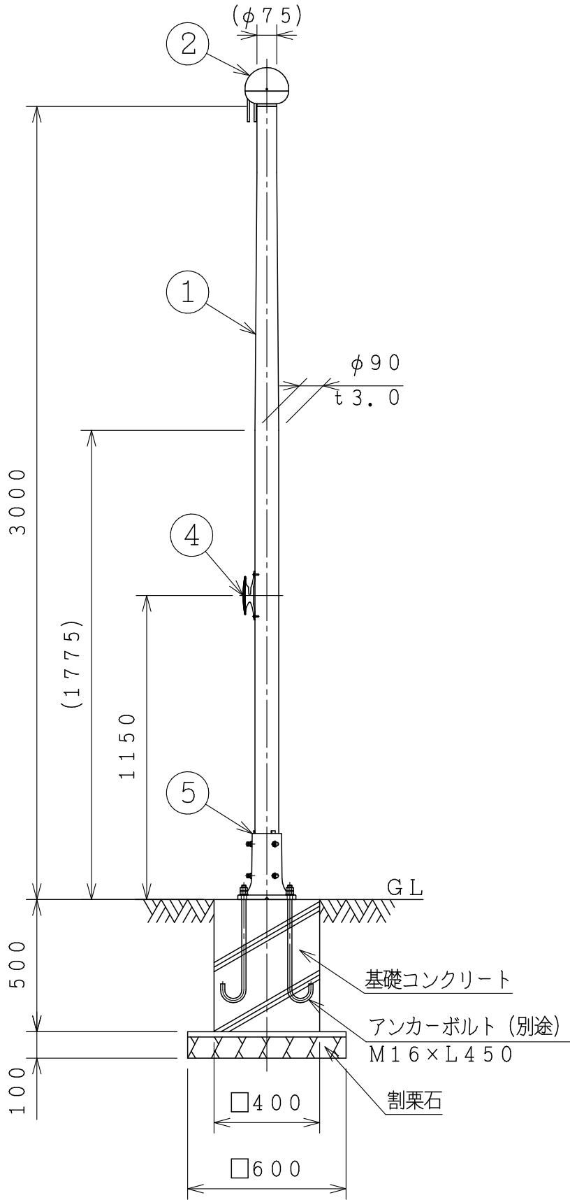
ポール姿図 S=1:20
