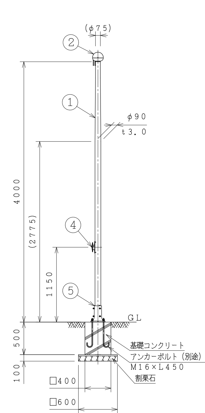
ポール姿図 S=1:30
