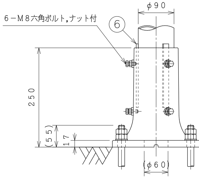
ベース部詳細 S=1:5
