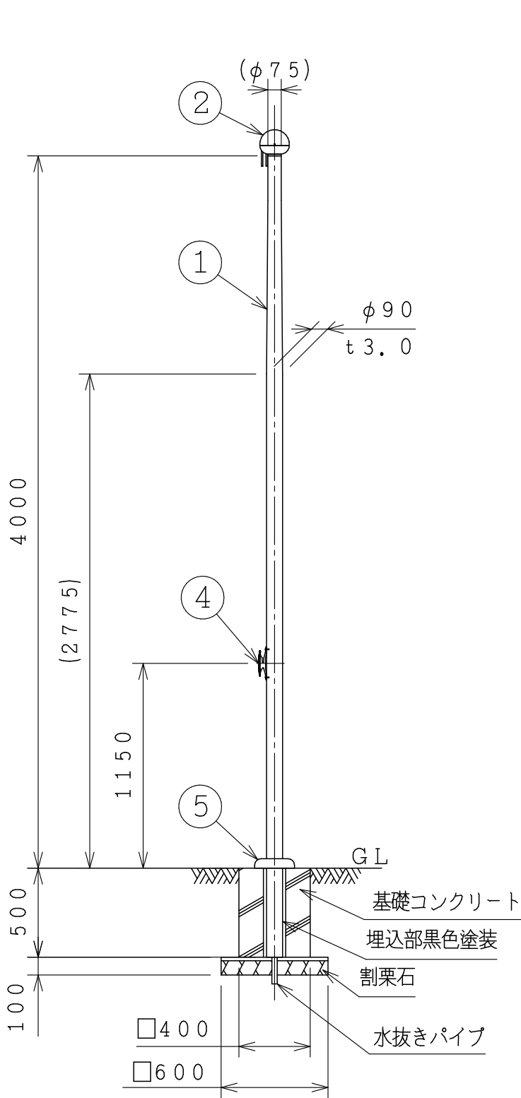
ポール姿図 S=1:30
