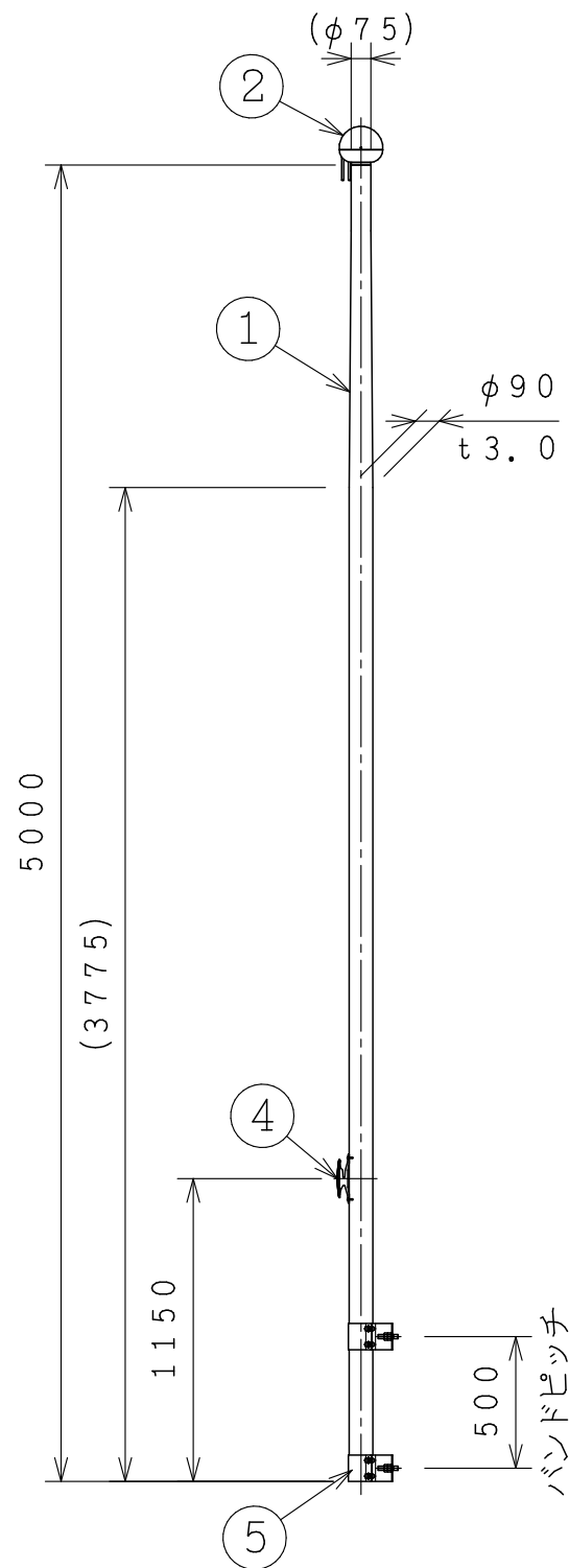
ポール姿図 S=1:30
