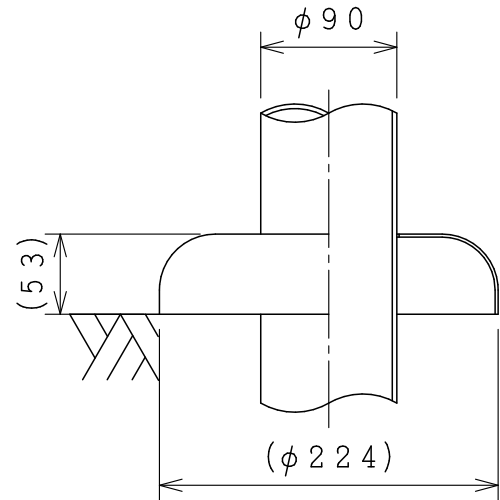
グランドカバー 詳細 S=1:5
