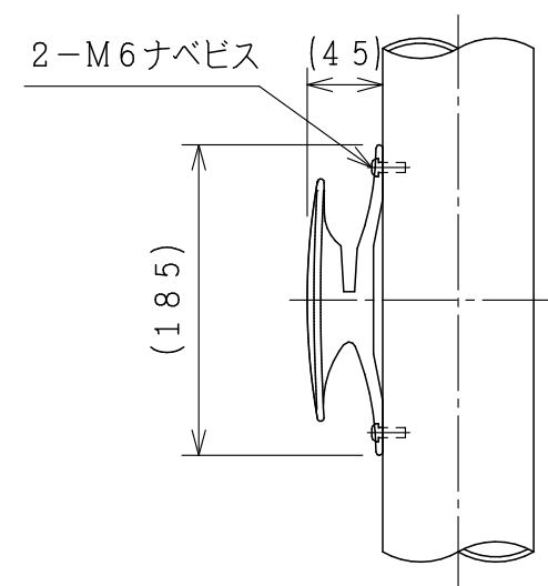
ロープ掛け部詳細 S=1:5
