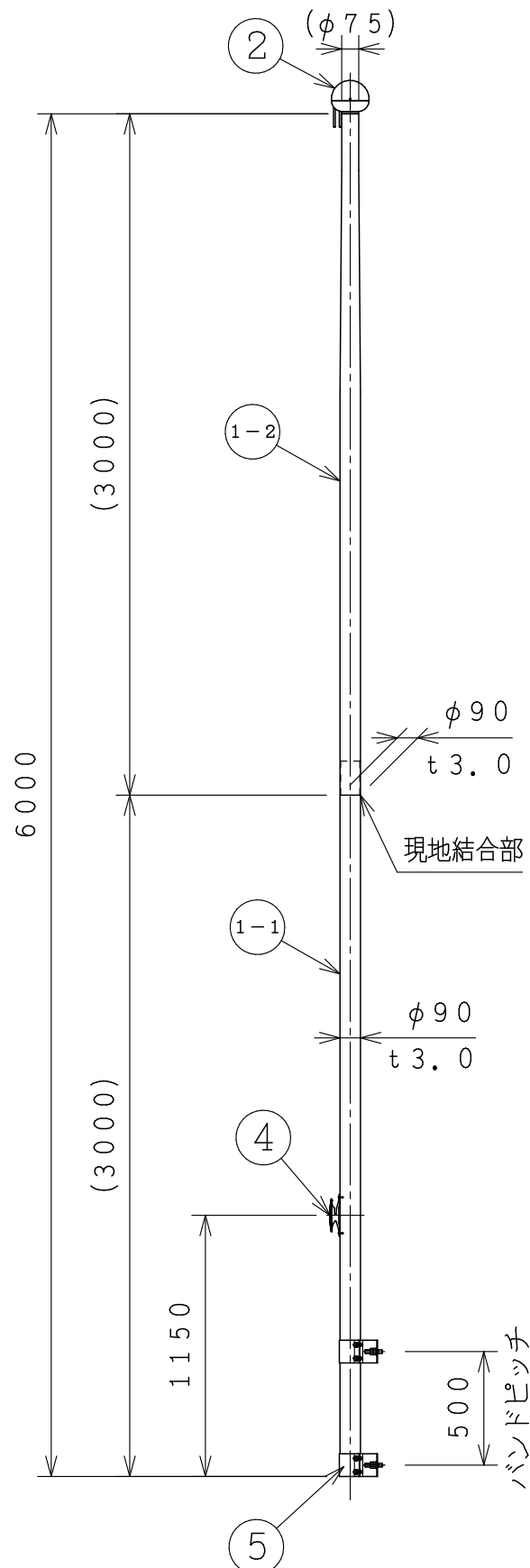
ポール姿図 S=1:30
