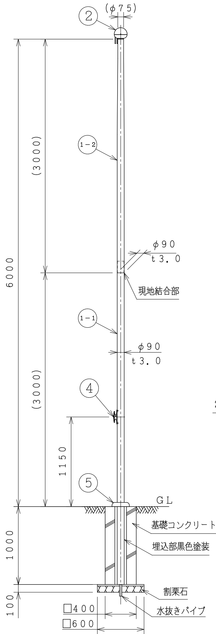
ポール姿図 S=1:30
