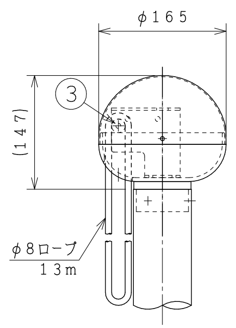
先端部詳細 S=1:5
