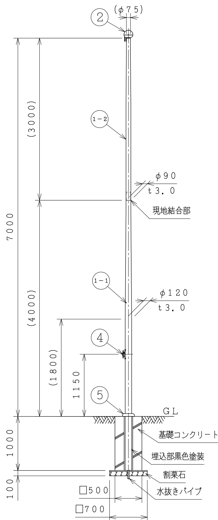
ポール姿図 S=1:40
