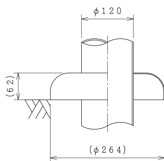
グランドカバー詳細 S=1:5
