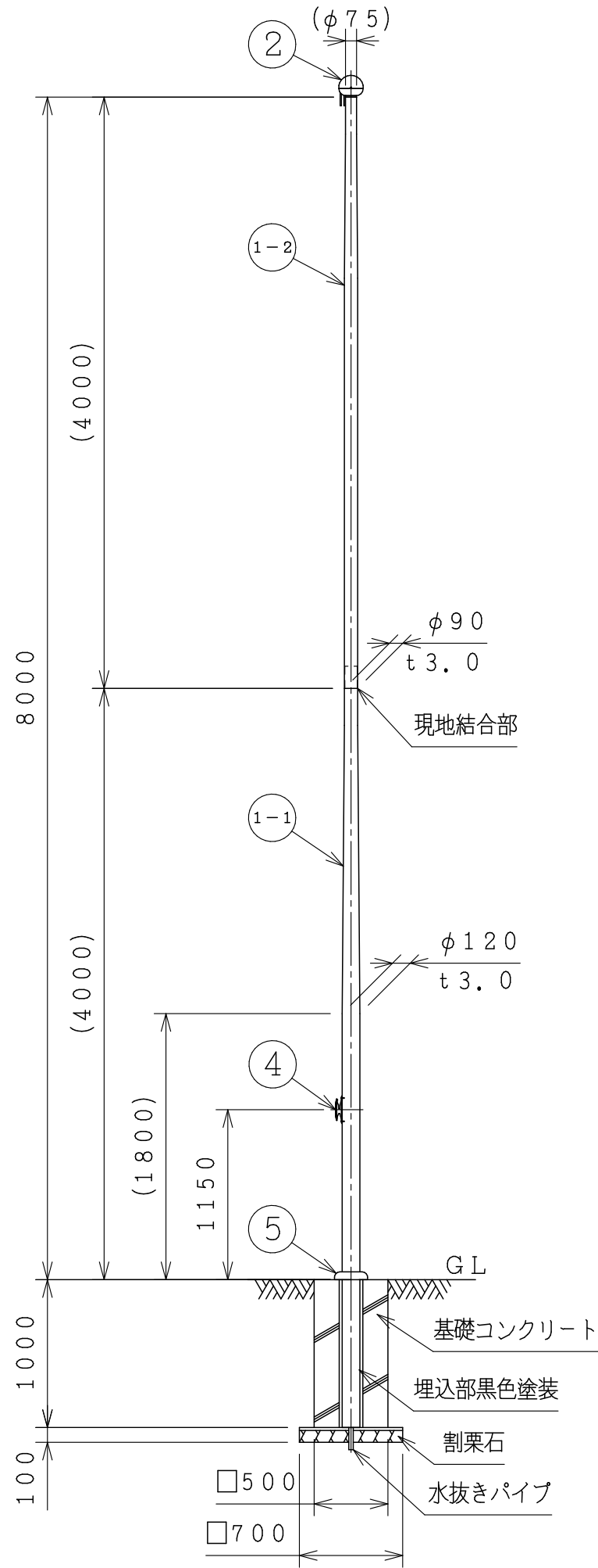
ポール姿図 S=1:40
