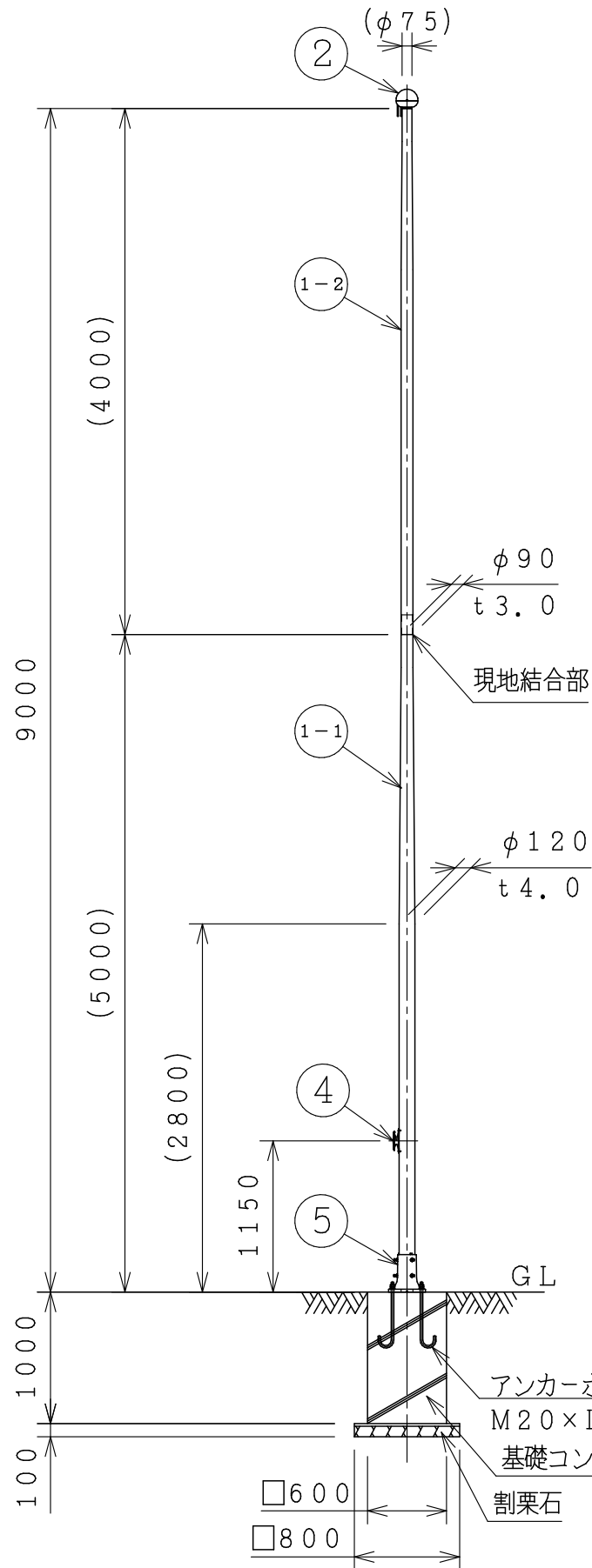
ポール姿図 S=1:50
