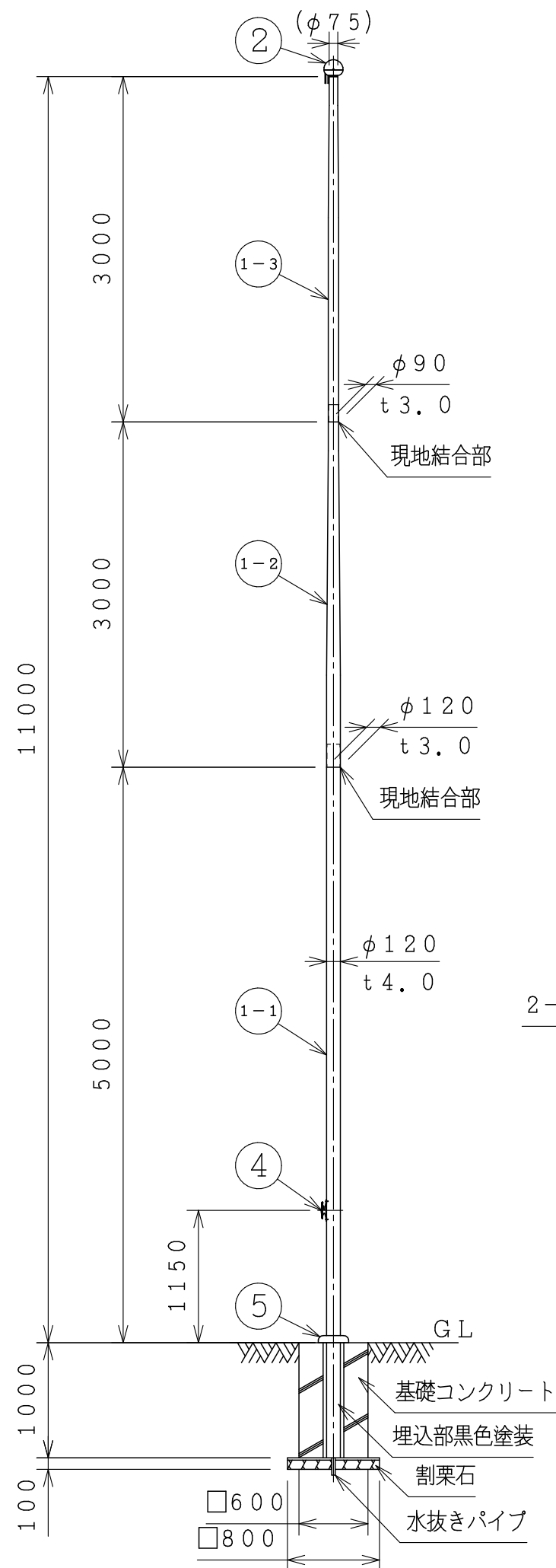
ポール姿図 S=1:50
