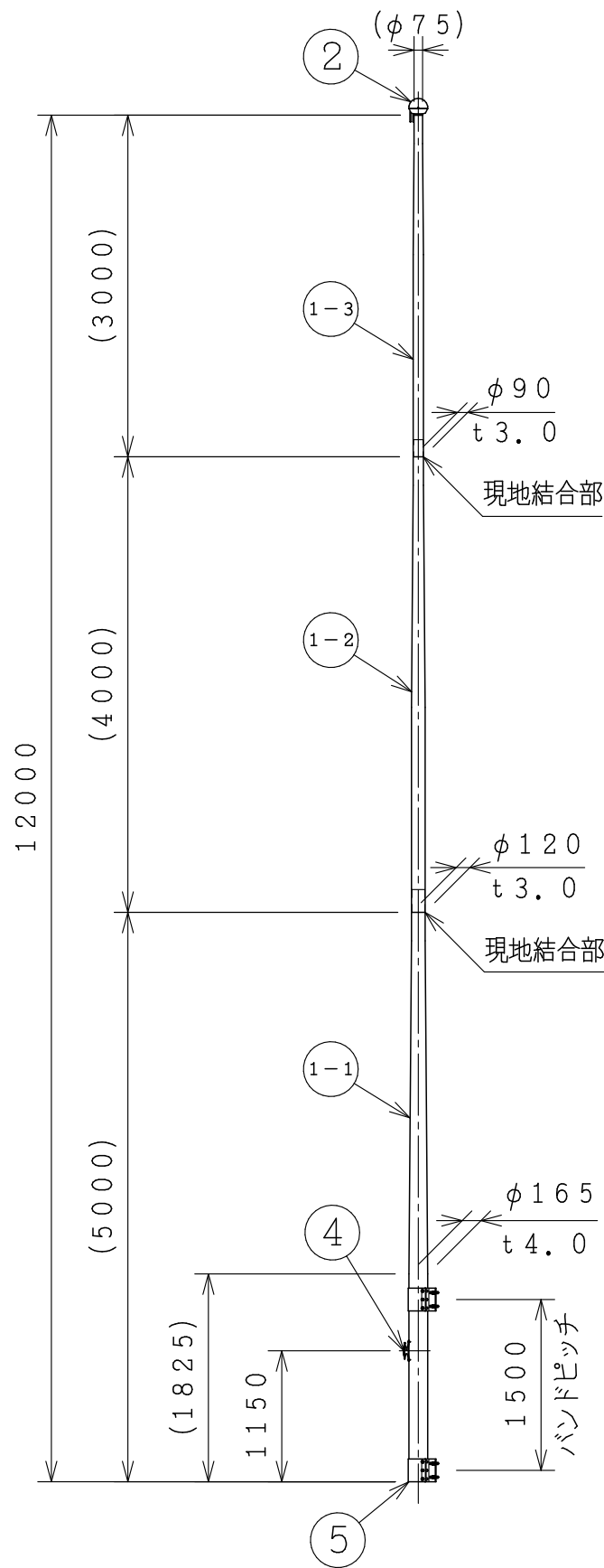
ポール姿図 S=1:60
