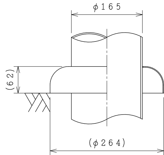
グラウンドカバー 詳細 S=1:5
