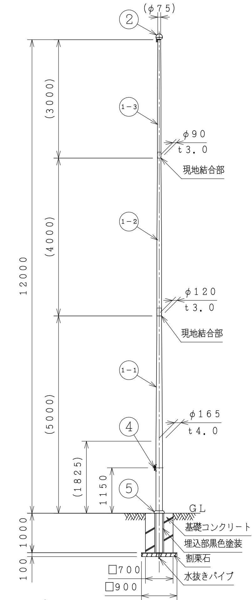
ポール姿図 S=1:60
