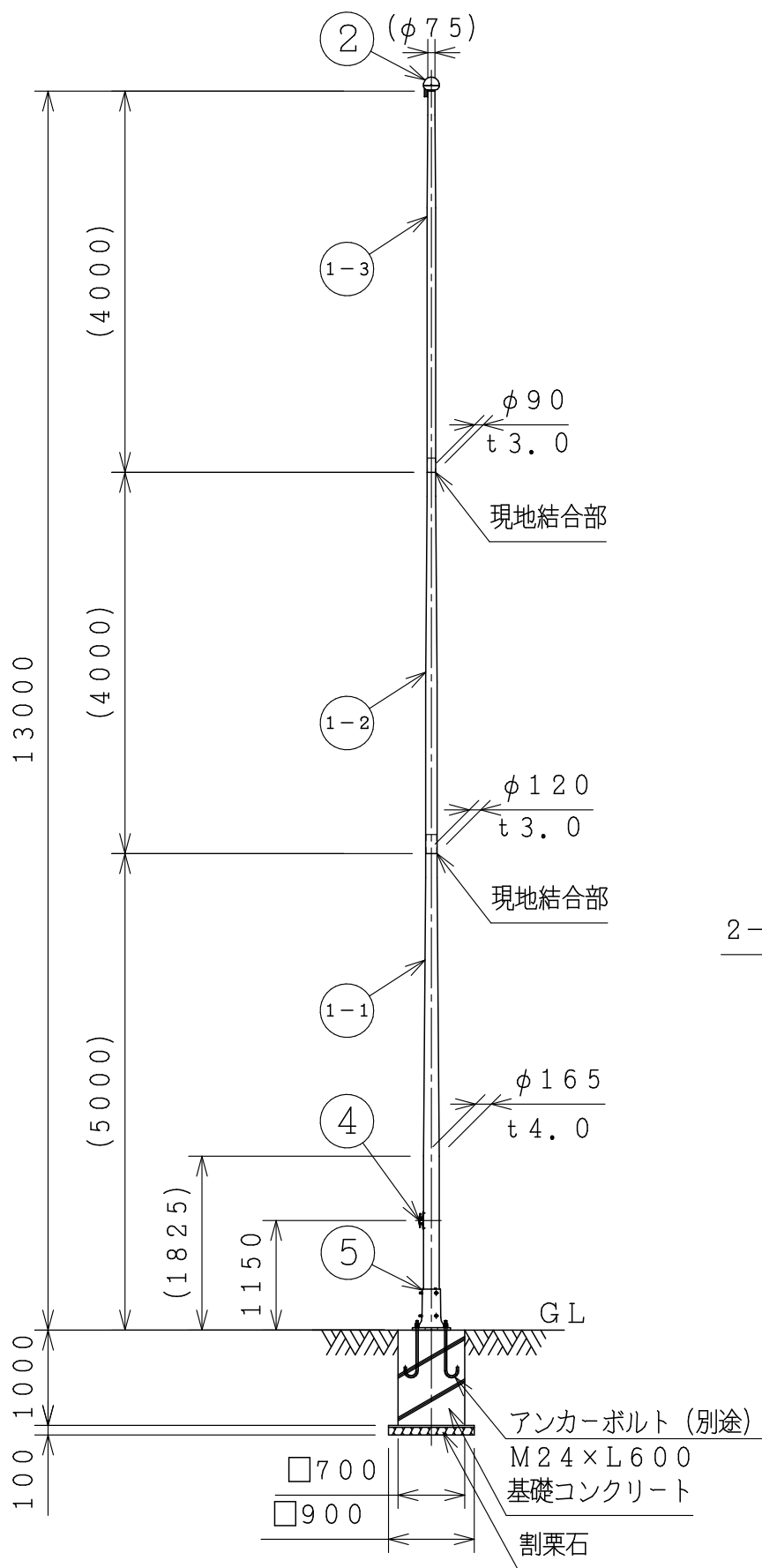
ポール姿図 S=1:70
