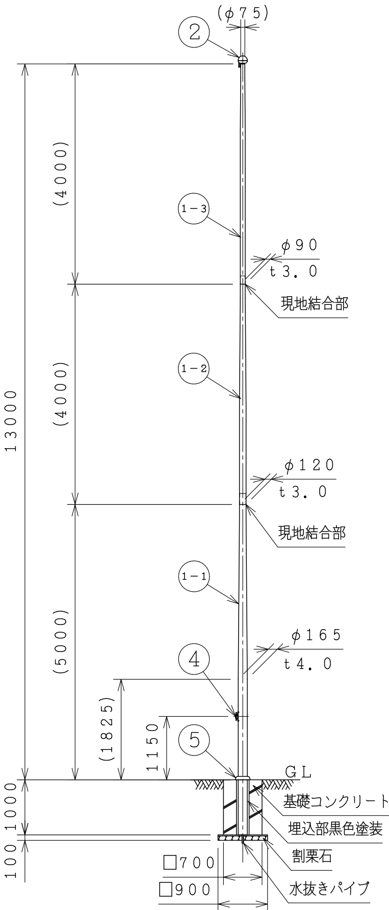
ポール姿図 S=1:70
