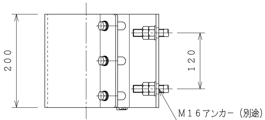
バンド部詳細
