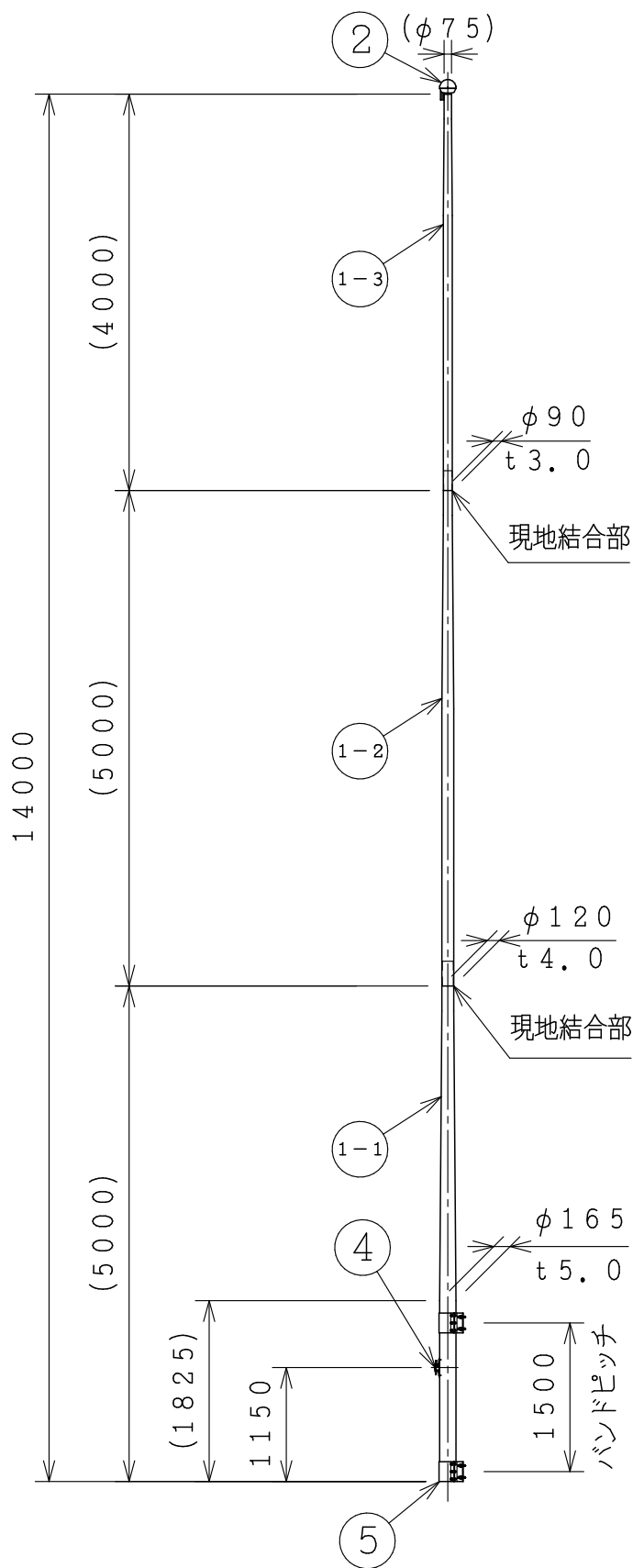
ポール姿図 S=1:70
