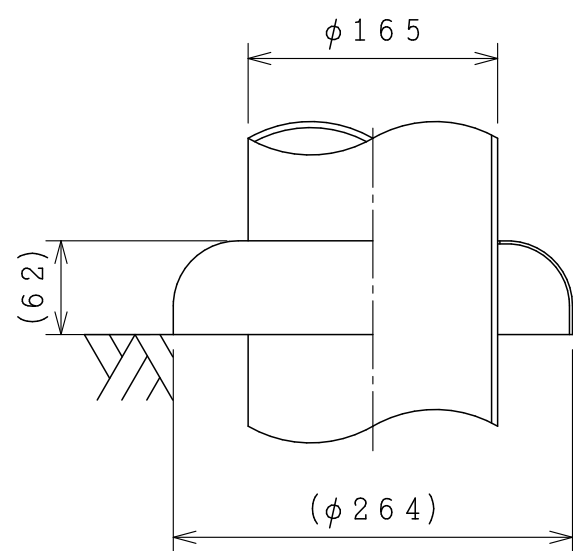
グランドカバー 詳細 S=1:5
