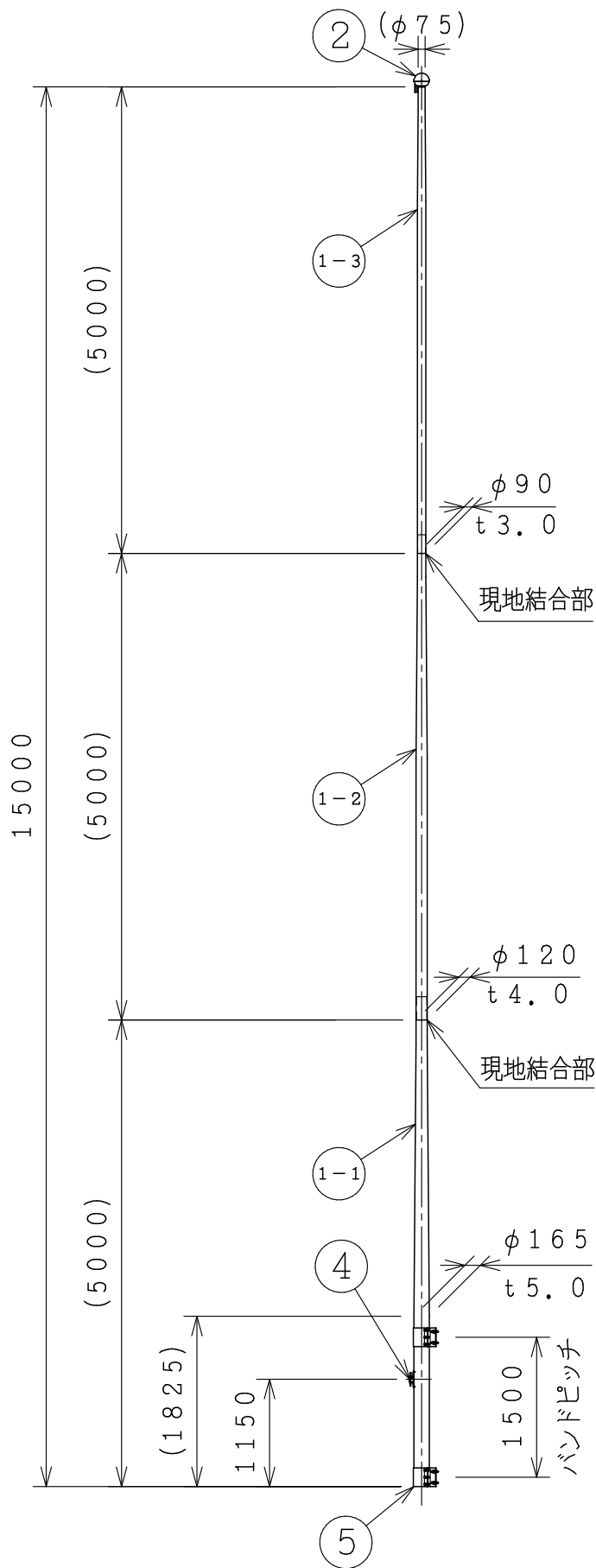
ポール姿図 S=1:70
