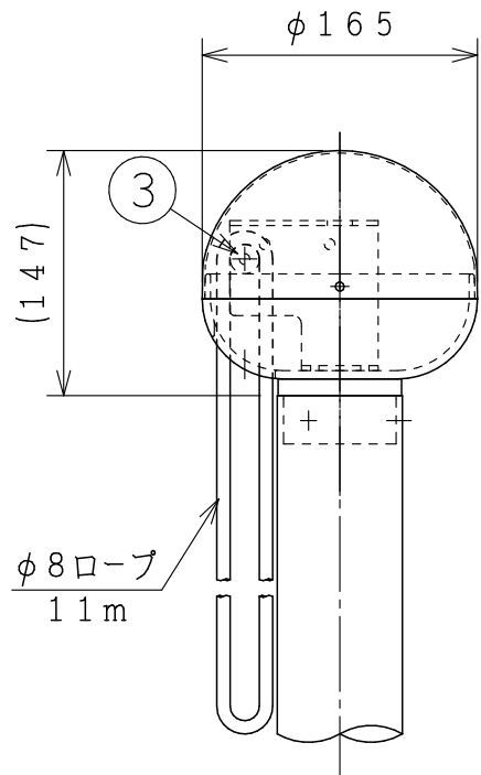
先端部詳細 S=1:5
