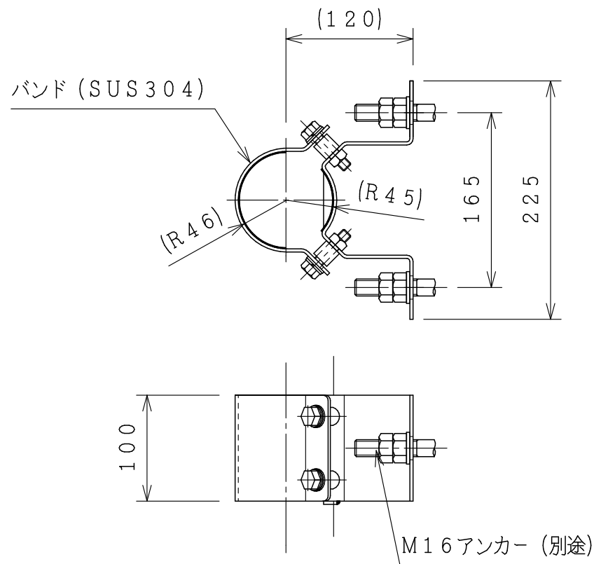
バンド部詳細 S=1:5
