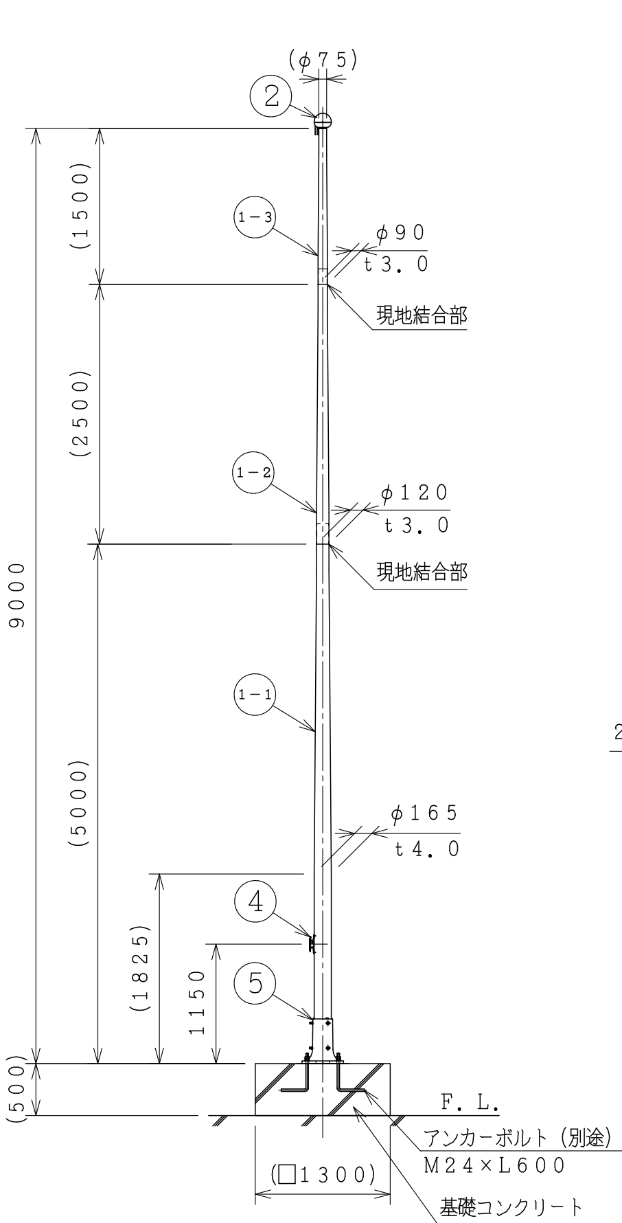
ポール姿図 S=1:50
