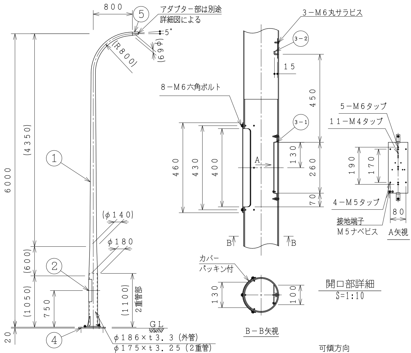
ポール姿図 S=1:40
