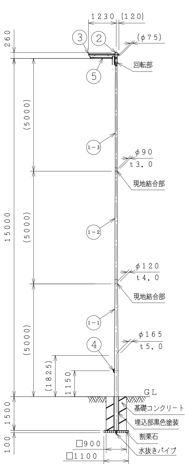
ポール姿図 S=1:80
